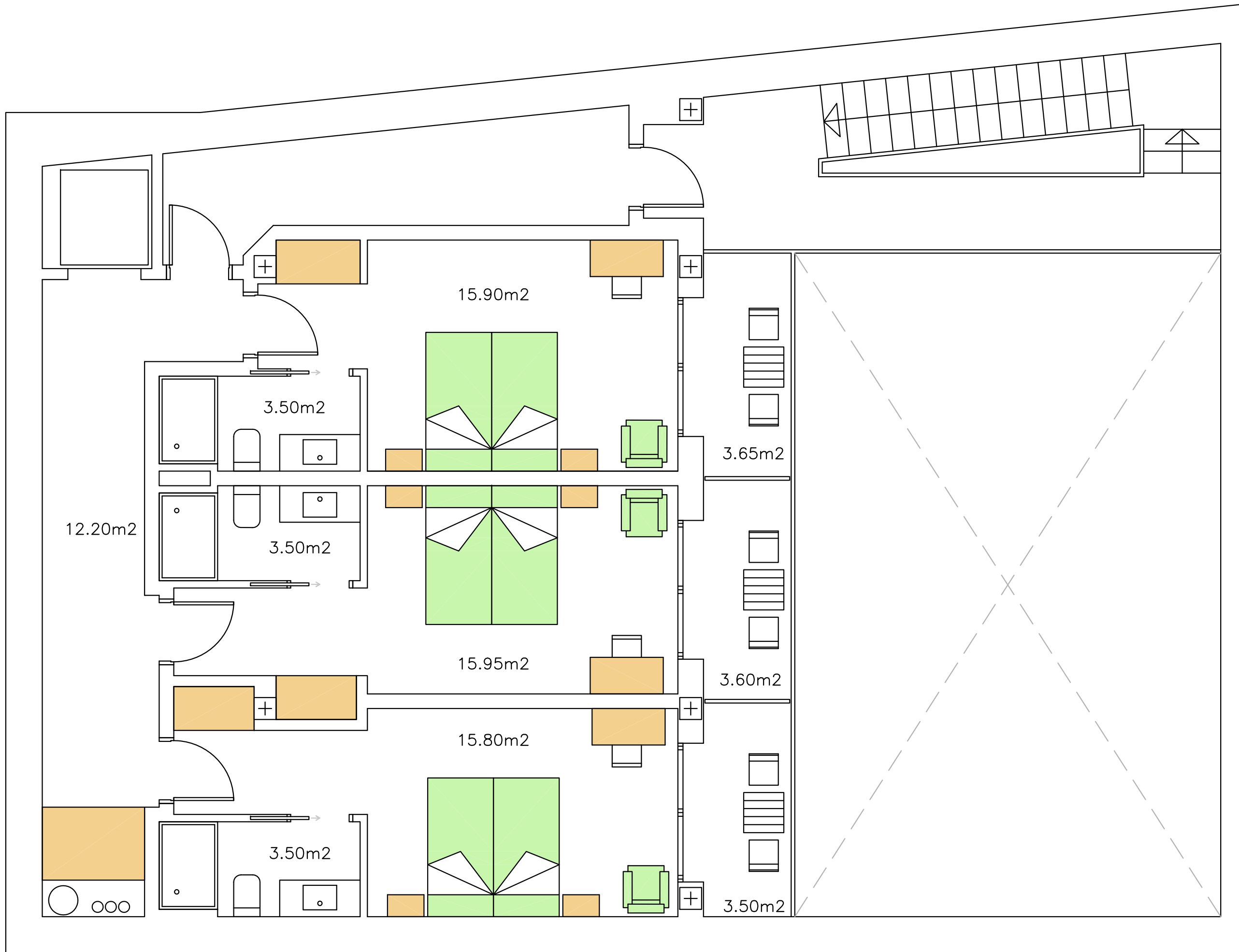
Planta pisos 1 i 2
